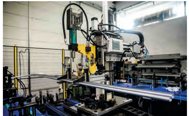
Robot di montaggio strutture metalliche porte sezionali. Robot for assembling metal structures for sectional doors.
